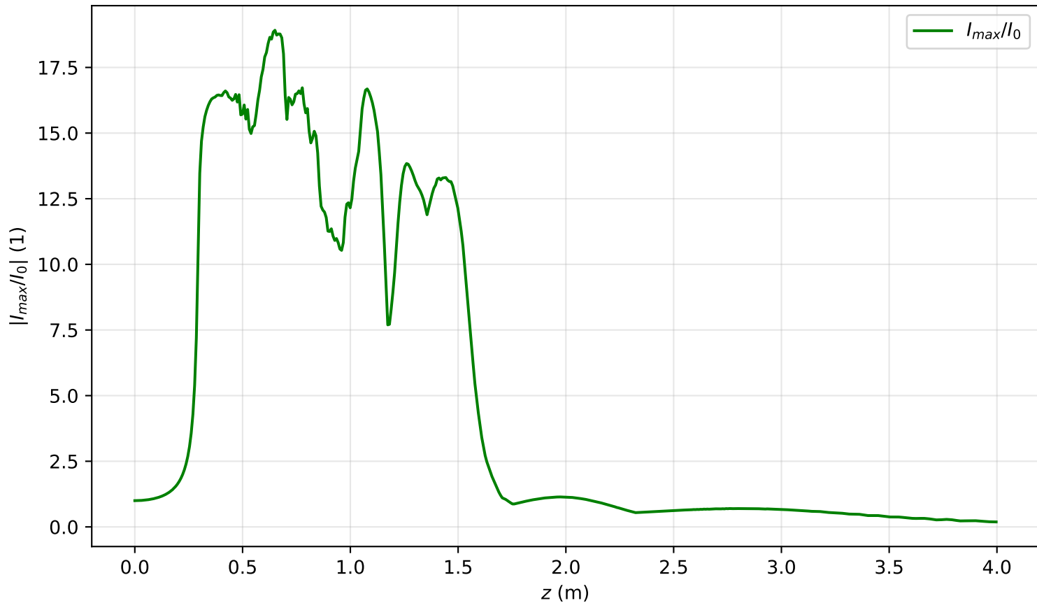
I_{\max}(r=0, z)/I_0 , Pin=9.5Pcr
